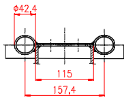
Ansicht X GLEITROHRFÜHRUNG
