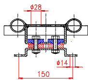
Ansicht Y WANDHALTERUNG
