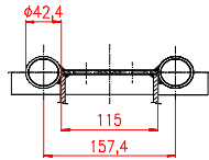
Ansicht Y WANDHALTERUNG
